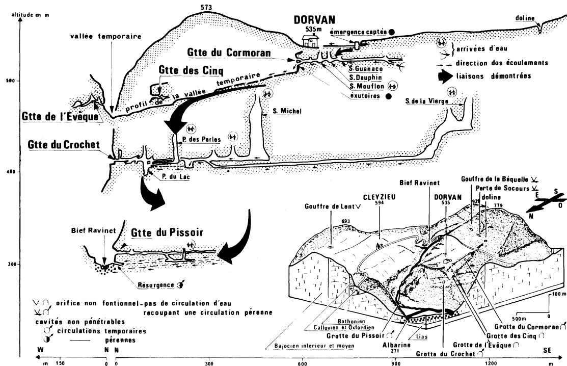
Fig. 11 - Complexe hydrogéologique de Dorvan : bloc-diagramme d'ensemble.
