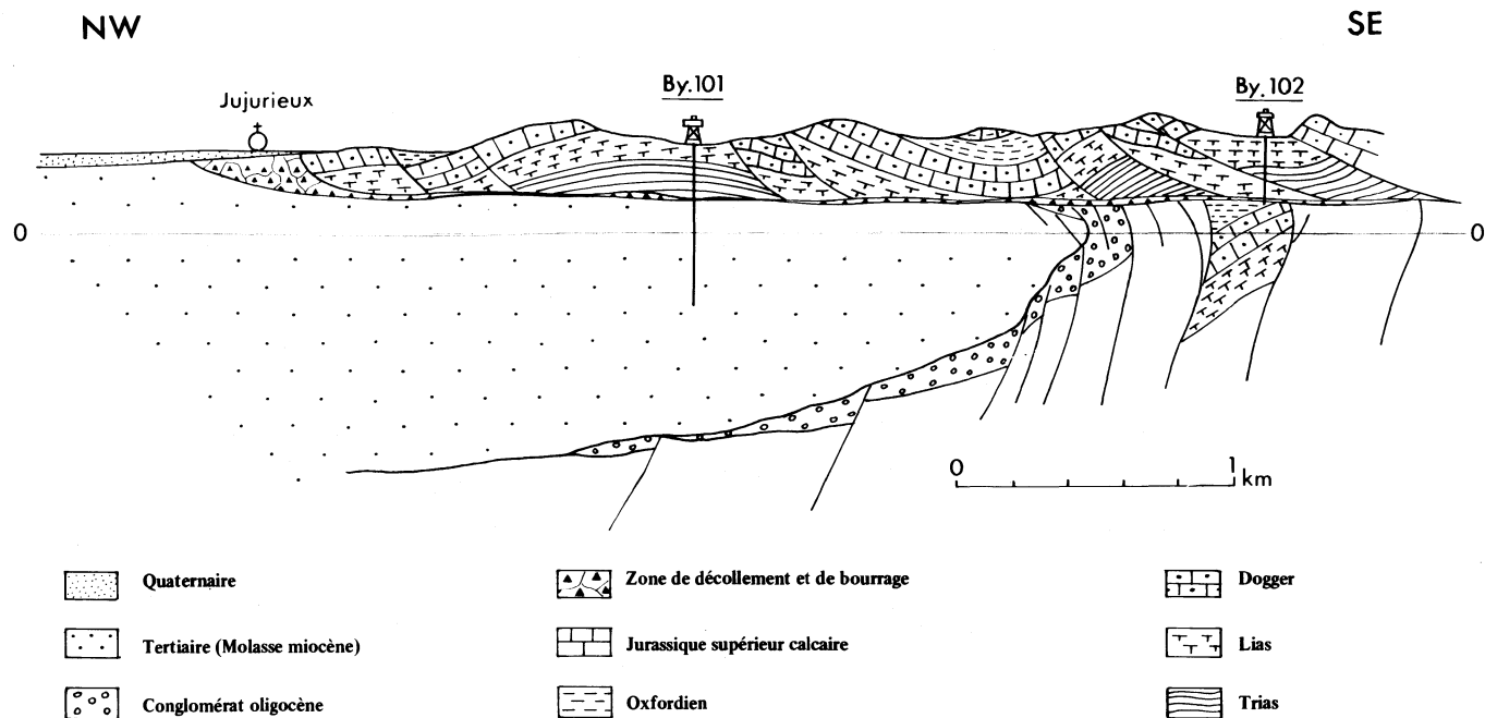
Fig. 10 - Contact Jura-Bresse et chevauchement frontal jurassien sur le fossé tertiaire
