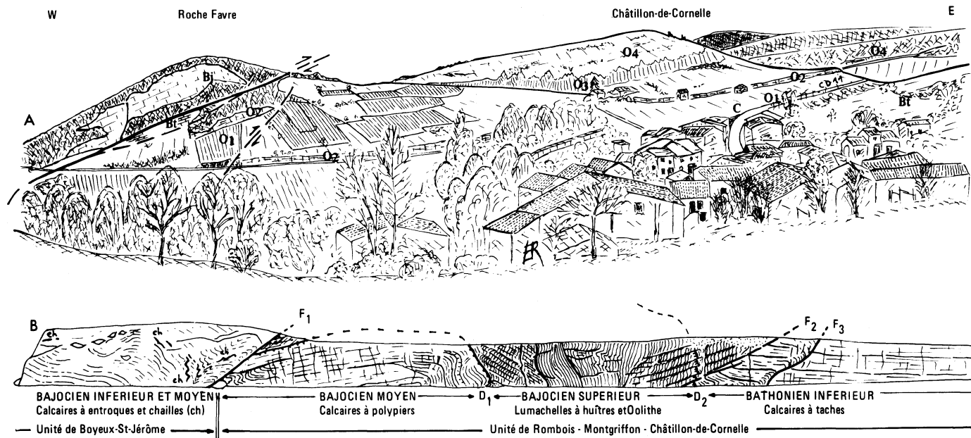
Fig. 9 - Affrontement entre l'unité de Boyeux-Saint-Jérôme ( à l'Ouest) et l'unité de Rombois-Montgriffon-Châtillon-de-Cornelle(à l'Est) dans la zone des lanières du faisceau bugiste
