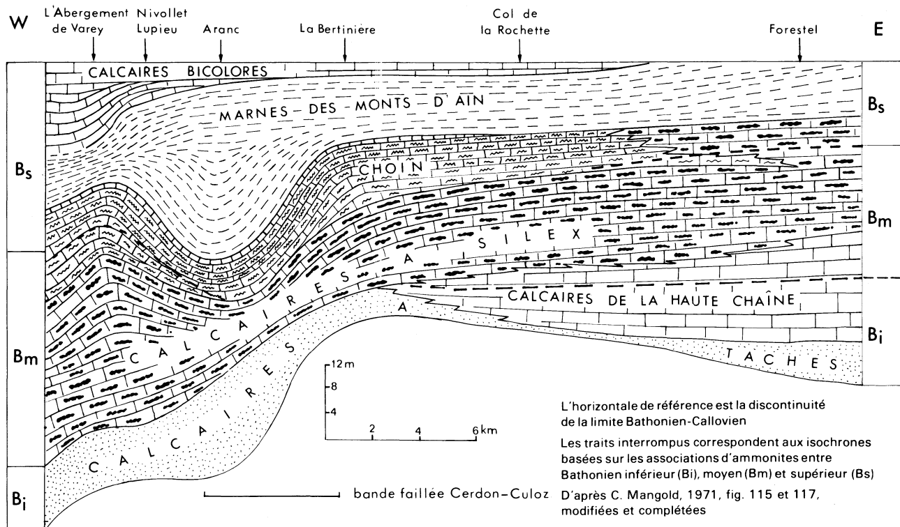
Fig. 3 - Section horizontale schématique (non dépliée) W-E, entre l'Abergement-de-Varey et le Grand-Colombier pour montrer les variations d'épaisseur et les relations entre les principales unités lithologiques du Bathonien sur la feuille Saint-Rambert-en-Bugey
