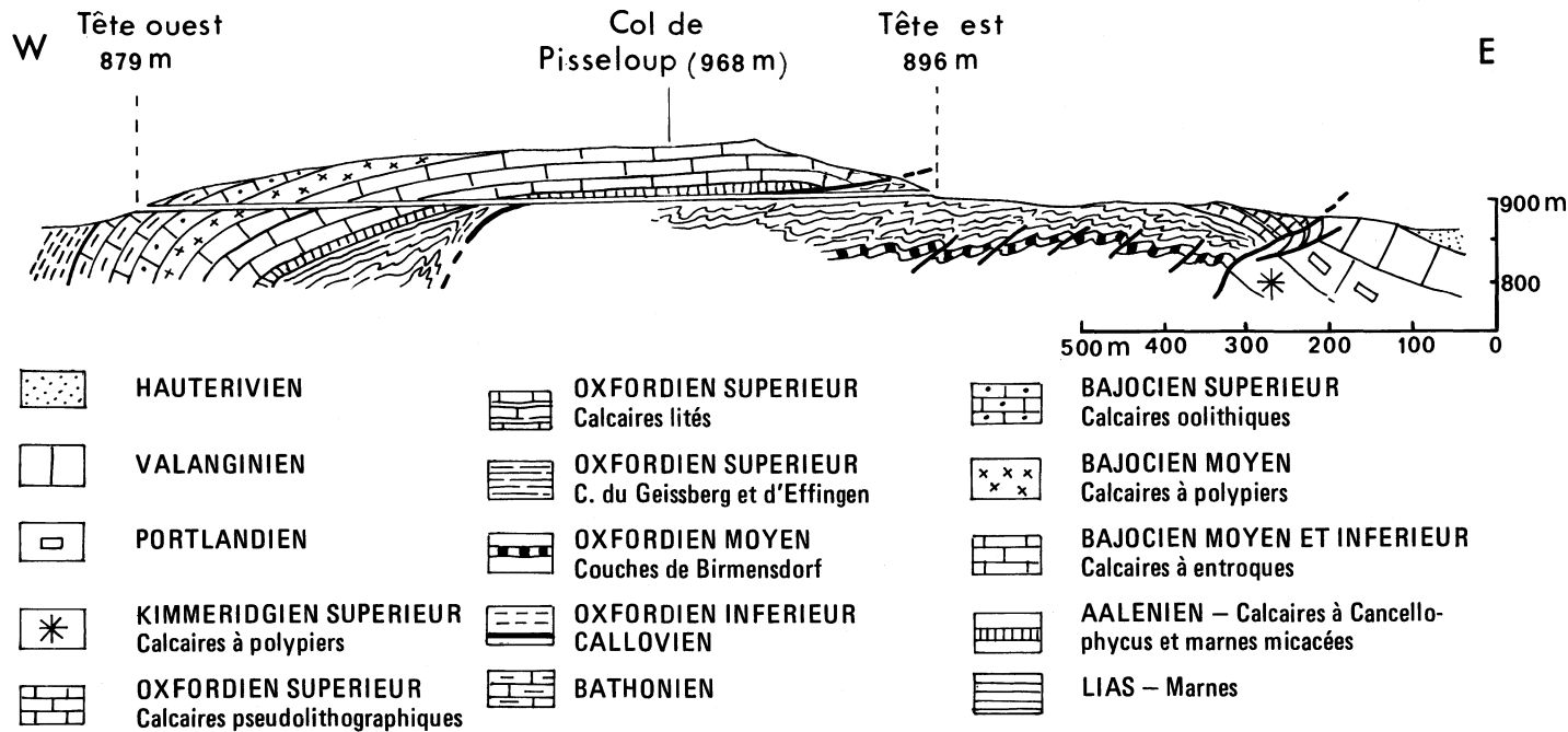
Fig. 8 - Accident-limite entre Jura externe et Jura interne et chevauchement (failles-plis) de l'anticlinal des monts d'Ain sur la lanière de Jurassique supérieur des Joux Blanches et sur le plateau d'Hauteville.
