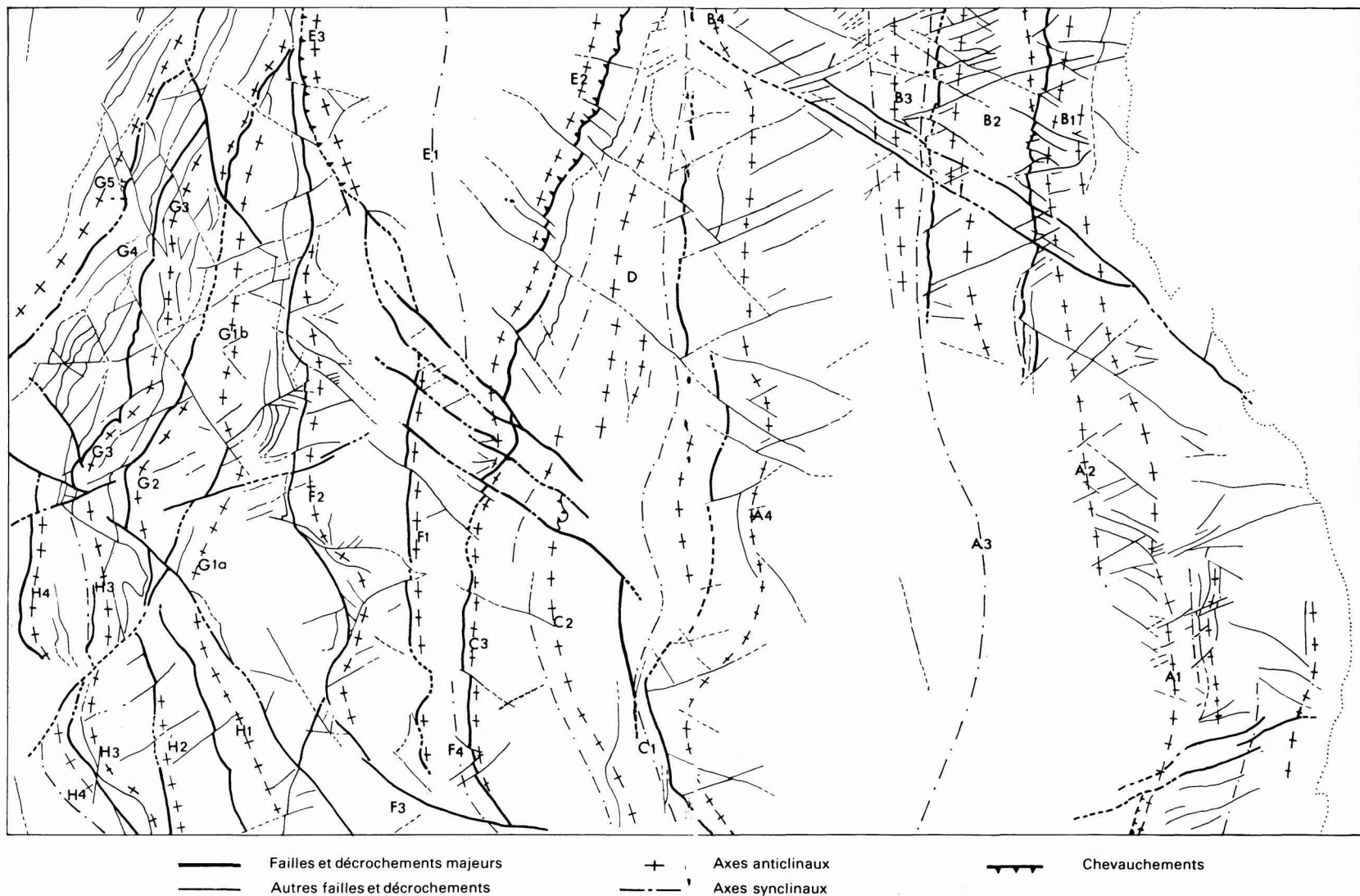
Fig. 6 - Schéma structural de la feuille Saint-Rambert-en-Bugey étendu à l'Est (Grand - Colombier) sur une partie de la feuille Seyssel
