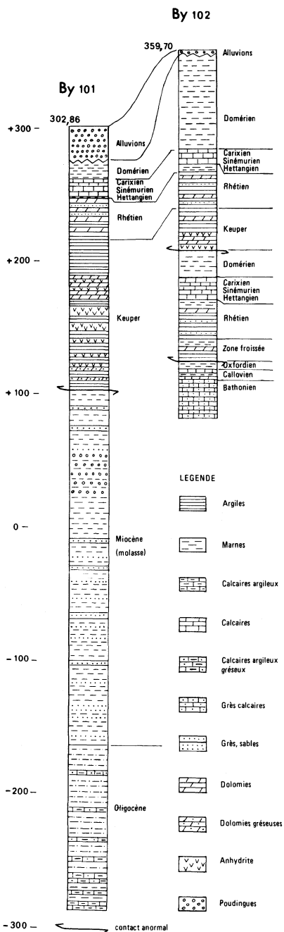
Fig. 13 - Coupes des sondages de reconnaissance d'hydrocarbures
